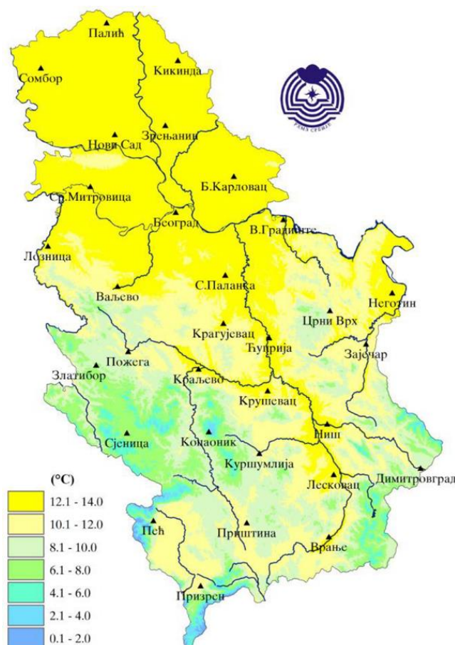
Слика 8.4. Средња температура ваздуха током пролећа 2019. године Picture 8.4. Mean air temperatures in the spring of 2019
