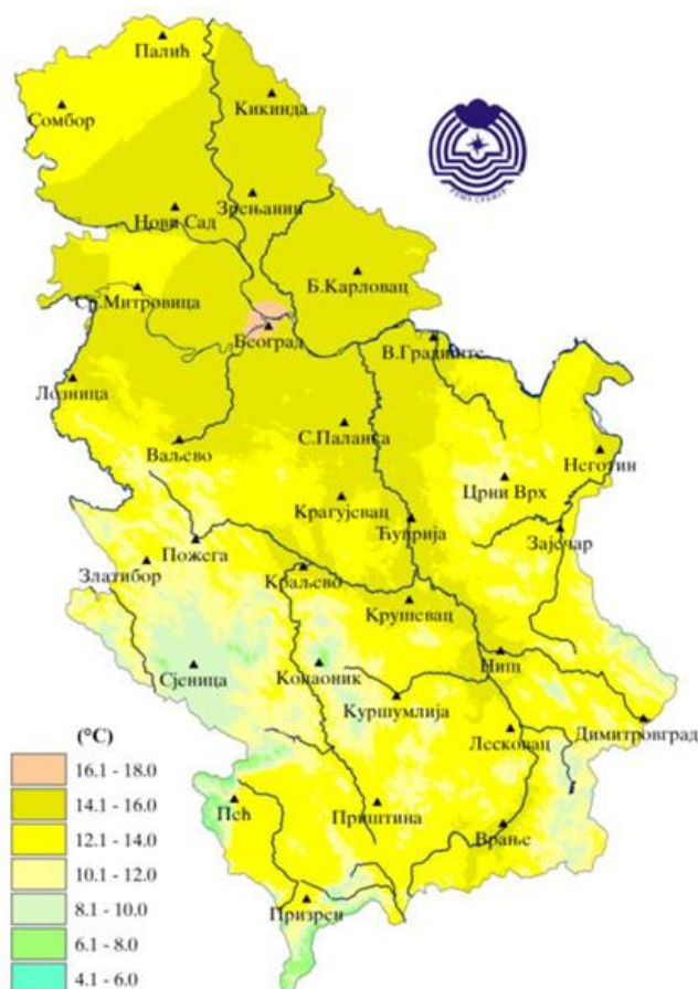
Слика 8.10. Средња температура ваздуха током јесени 2019. године Picture 8.10. Mean air temperatures in the autumn of 2019
